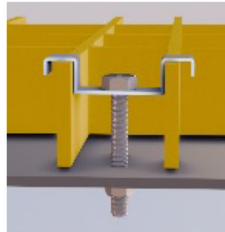
M-Clip
